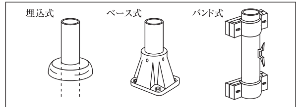
図2. 根元詳細
