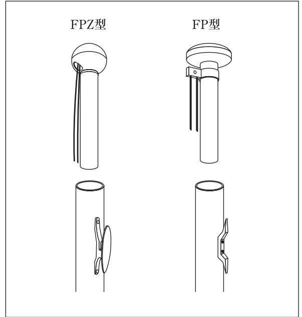
図1. ポール
