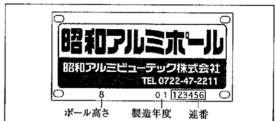
図3. 銘板
